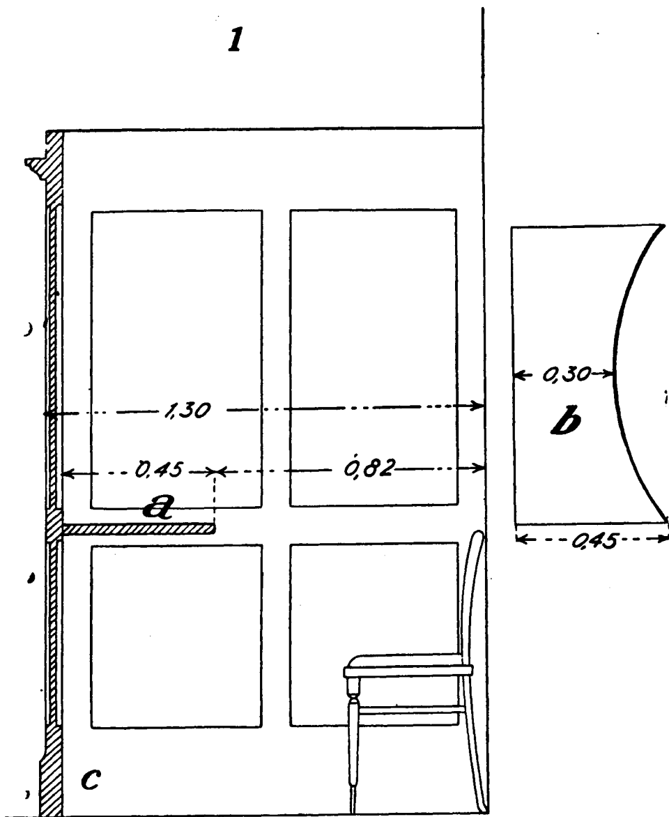
1. Prospetto del tavolo senza schermo verso l'Ufficio
